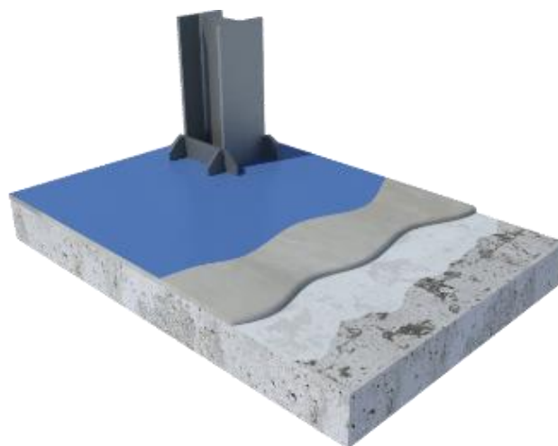
Figura 1.1: Representación esquemática del sistema de pavimentación.
