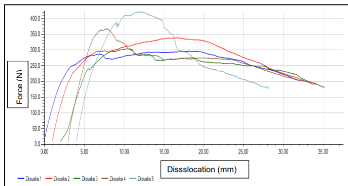
Figura A4.3: Gráfico carga/desplazamiento del ensayo de atravesamiento de webertherm placa DUO (TR 7,5) con un espesor de 50 mm en condiciones secas cuando las fijaciones están situadas en el cuerpo del aislante y la arandela tiene una rigidez \geq 0,6 kN/mm.
