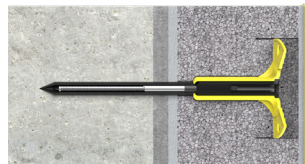
Detalle 4.1b Instalación avellanada
