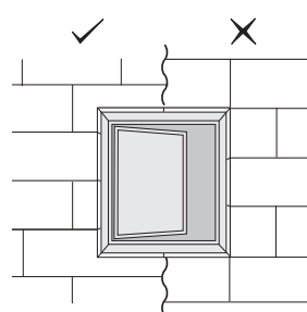
Detalle 3b Instalación de las placas de aislamiento en los cantos de esquina de un hueco.
