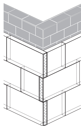
Detalle 3a Instalación de las placas de aislamiento en las aristas del edificio.
